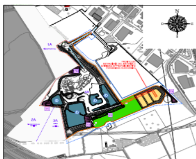
FASE 2 ESTRAZIONE NEL SETTORE EST DELL'AMPLIAMENTO
