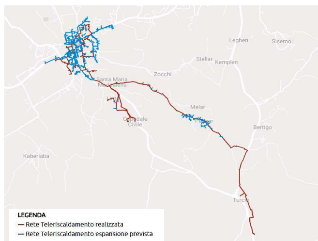
Rete di teleriscaldamento alimentata da centrale a biomassa Comune di Asiago
